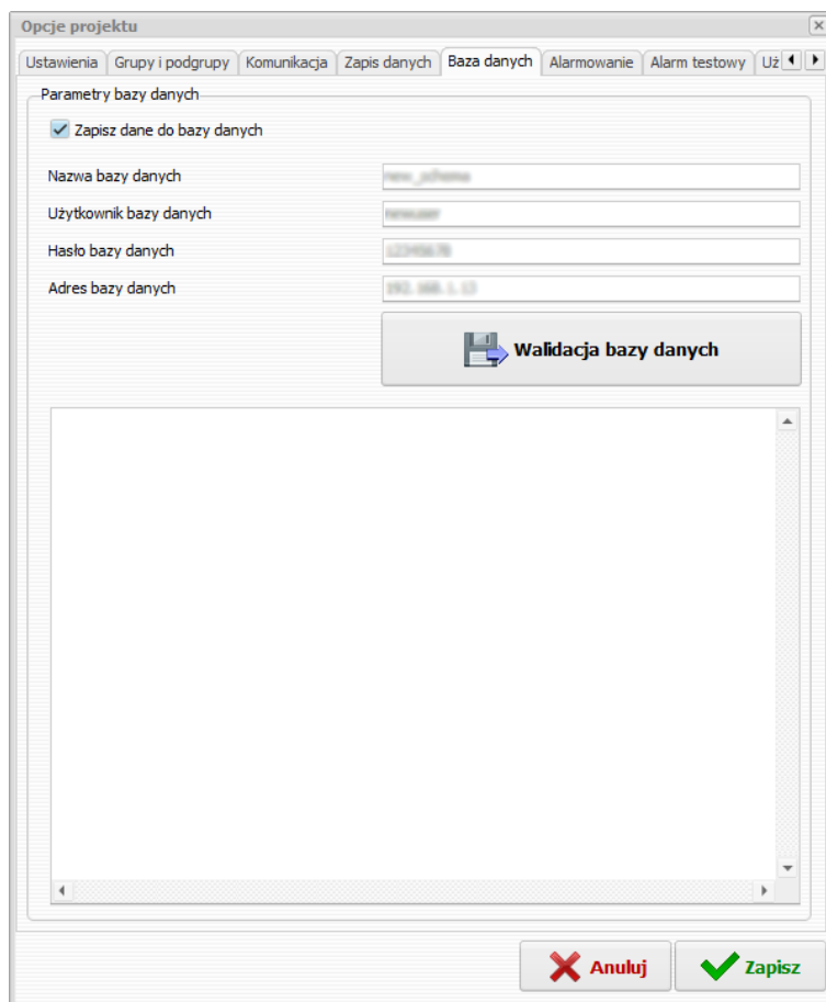
Rys. 1. Opcje projektu – zakładka Baza danych
